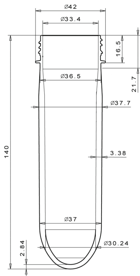
A-A View/Görünüm
